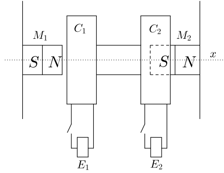
Fig. 46: Generator
