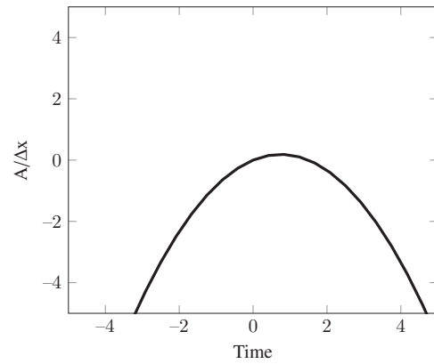
Fig. 4: A/Δx function
