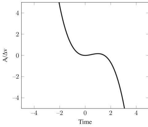
Fig. 5: A/Δv function
