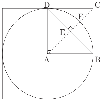
Fig. 45: Internal tangent circle
