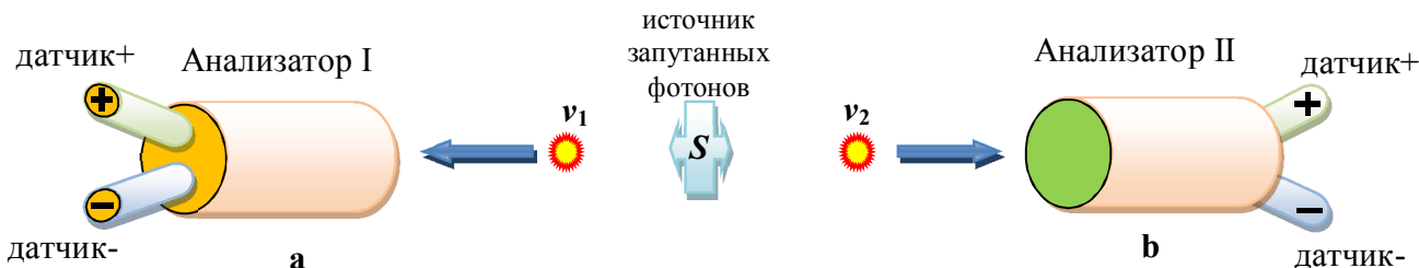
Рис.2 Мысленный эксперимент Эйнштейна-Подольского-Розена с фотонами (подобие схемы, взятой из работы Аллена Аспекта). Два фотона \nu_1 и \nu_2 , испускаемые источником S , проанализированы линейными поляризаторами в направлениях \mathbf{a} и \mathbf{b} .
